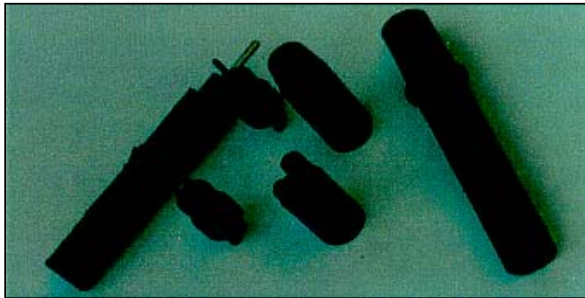
ŞEKİL 3 : Primer ve sekonder fiş ve prizler (ekransız kablo için)
