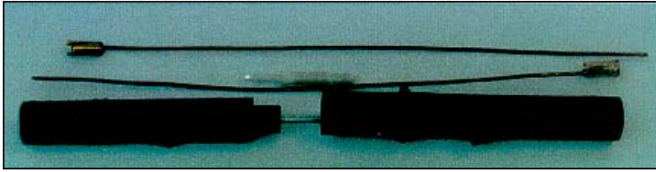
ŞEKİL 1 : Primer fiş ve priz (ekranlı kablo için) montajdan önce
