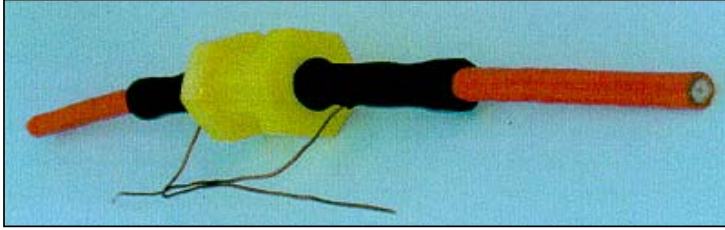
ŞEKİL 2 : Primer fiş ve priz (ekranlı kablo için) montajı tamamlanmış
